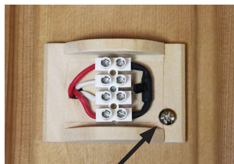
1 Stk. PH 3,5 x 17 mm
